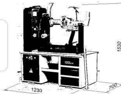
Net weight : 394 kg ( without lathe ) Net ağırlık : 394 kg ( tornasız )
