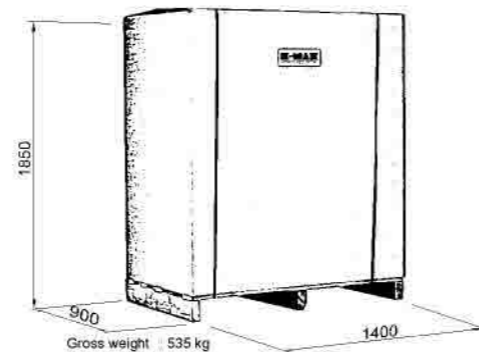
Gross weight 535 kg Brüt ağırlık 535 kg
